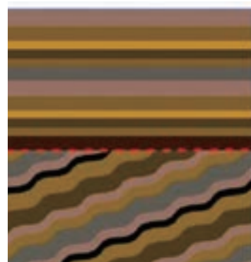
前弧海盆堆積体 不整合面 付加体
