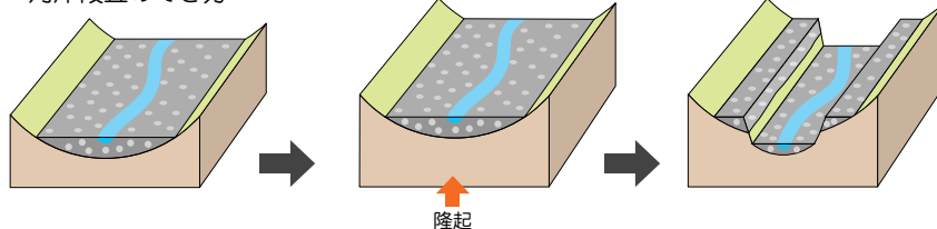
河岸段丘のでき方
